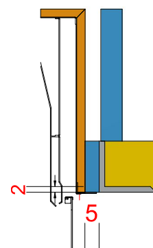
E) Variante poutre sans linteau
