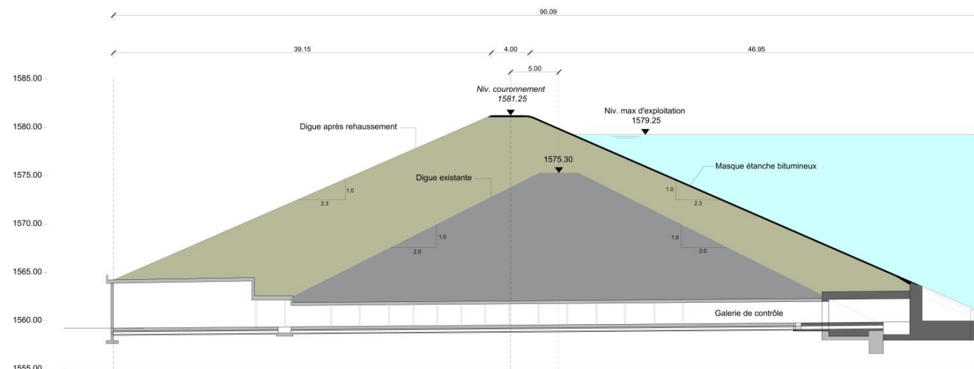
Coupe de principe de la digue (CORDONIER & REY SA)
